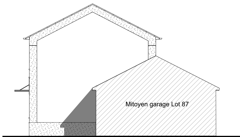
Pignon DROIT
