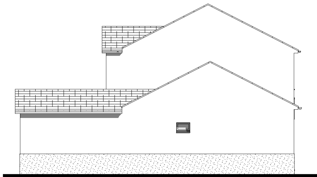
Pignon DROIT
