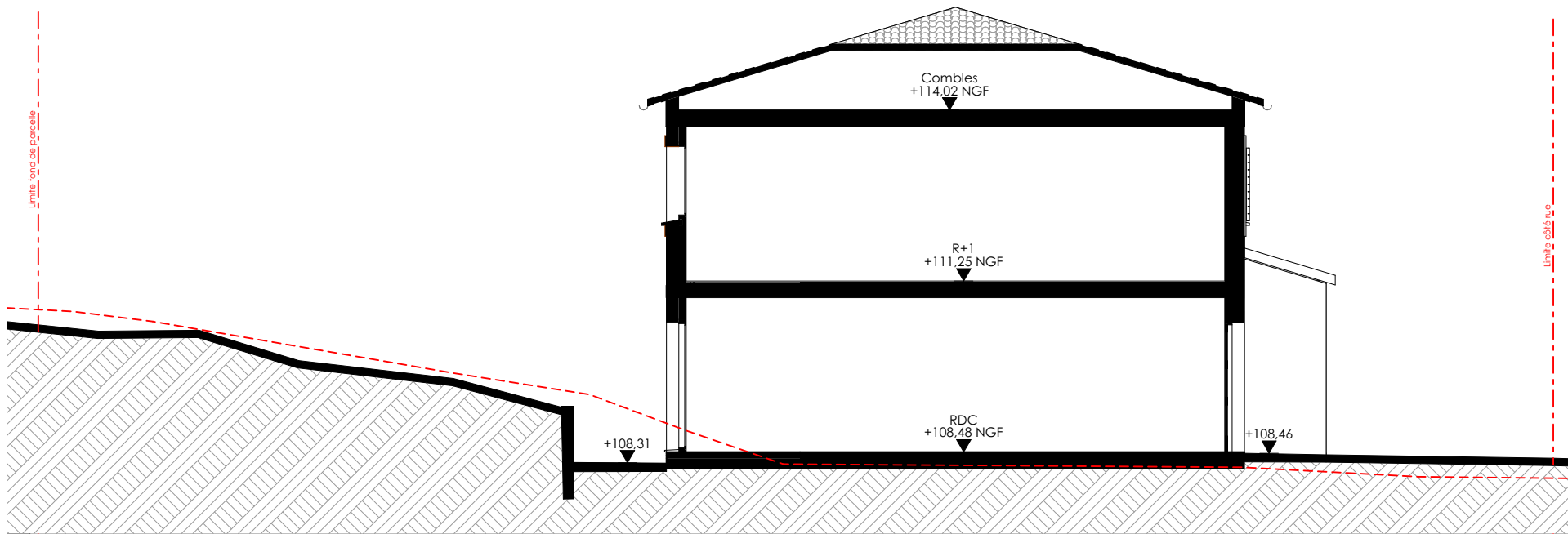
Coupe AA
