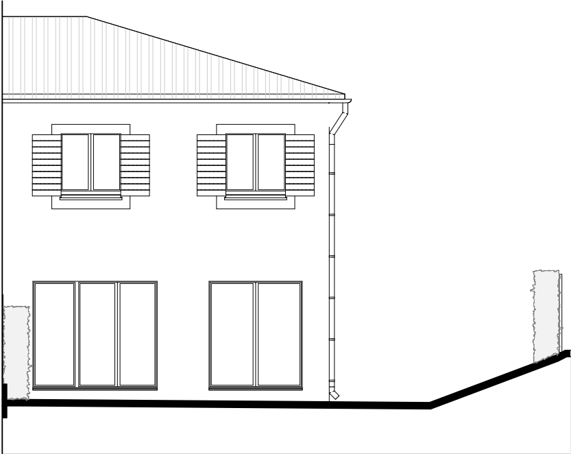
Façade Sud
