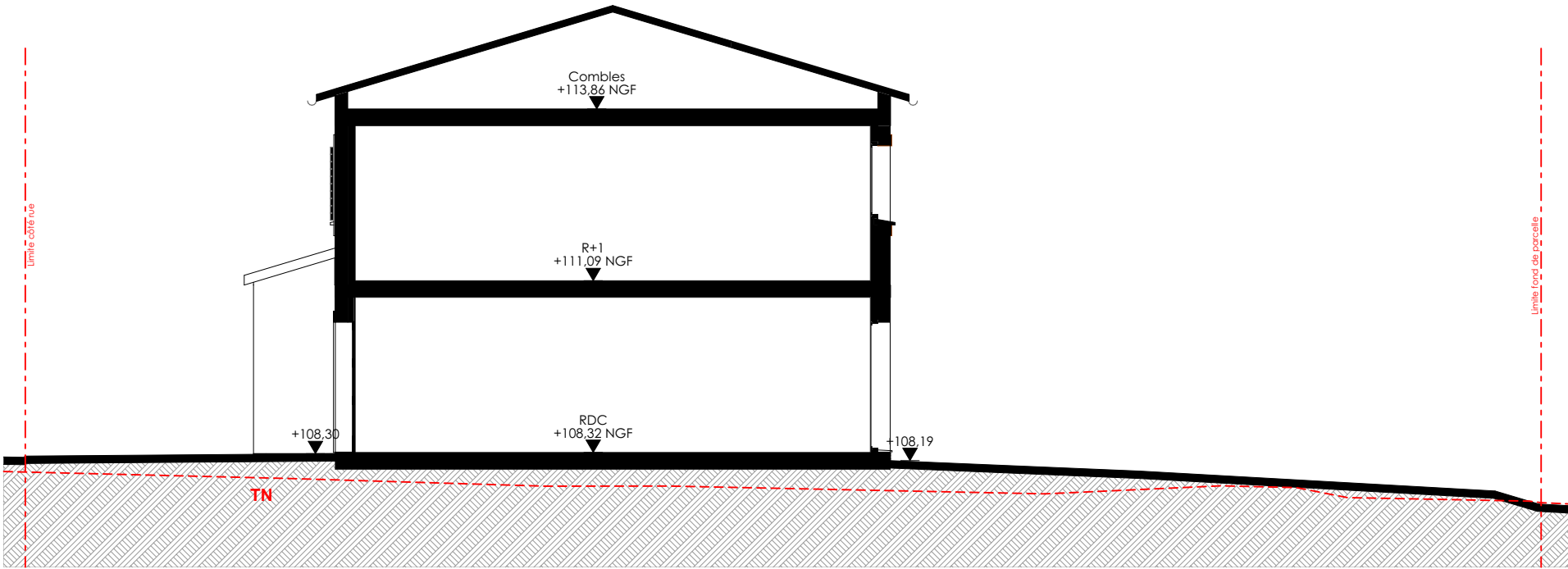
Coupe AA
