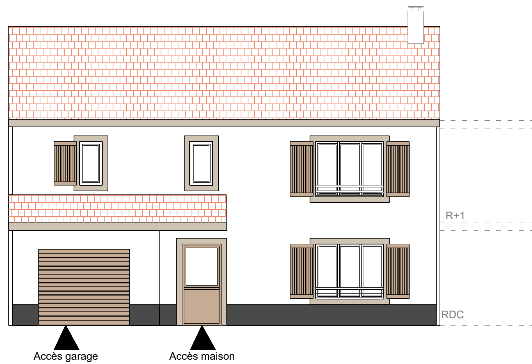
Façade AVANT
