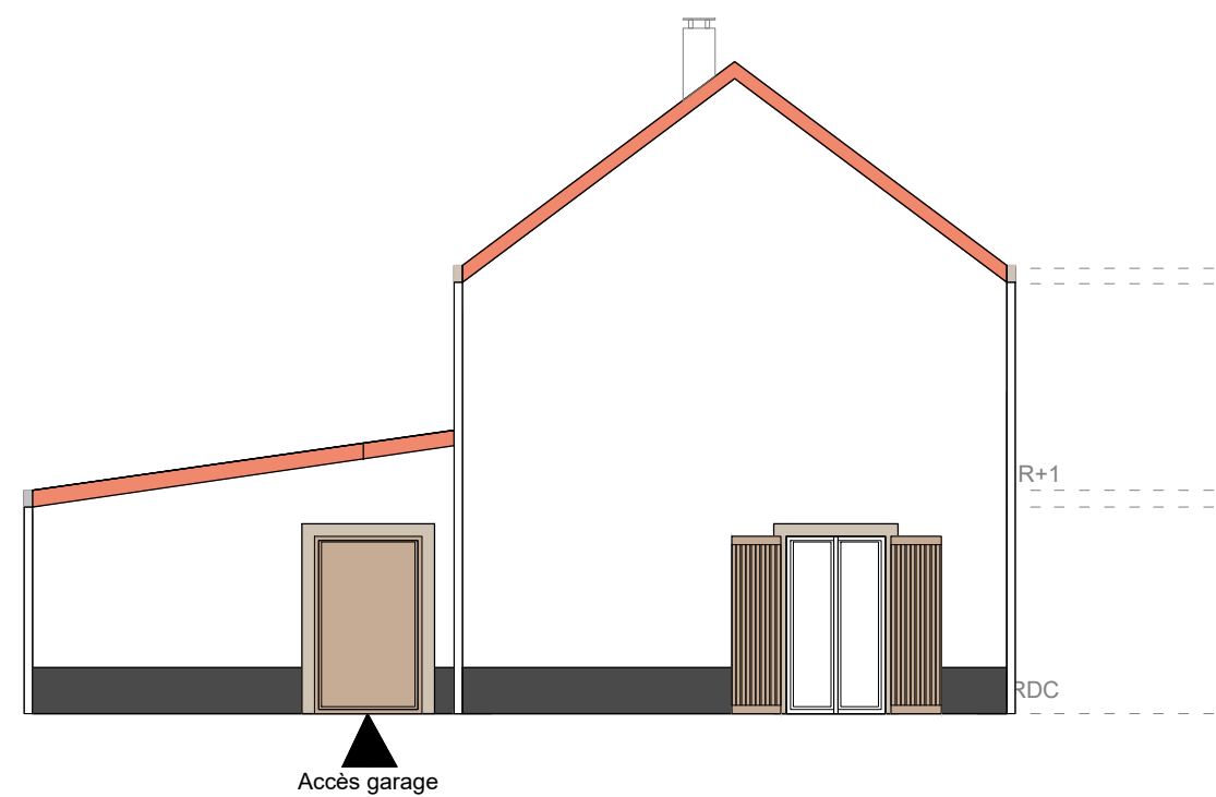
Pignon DROIT
