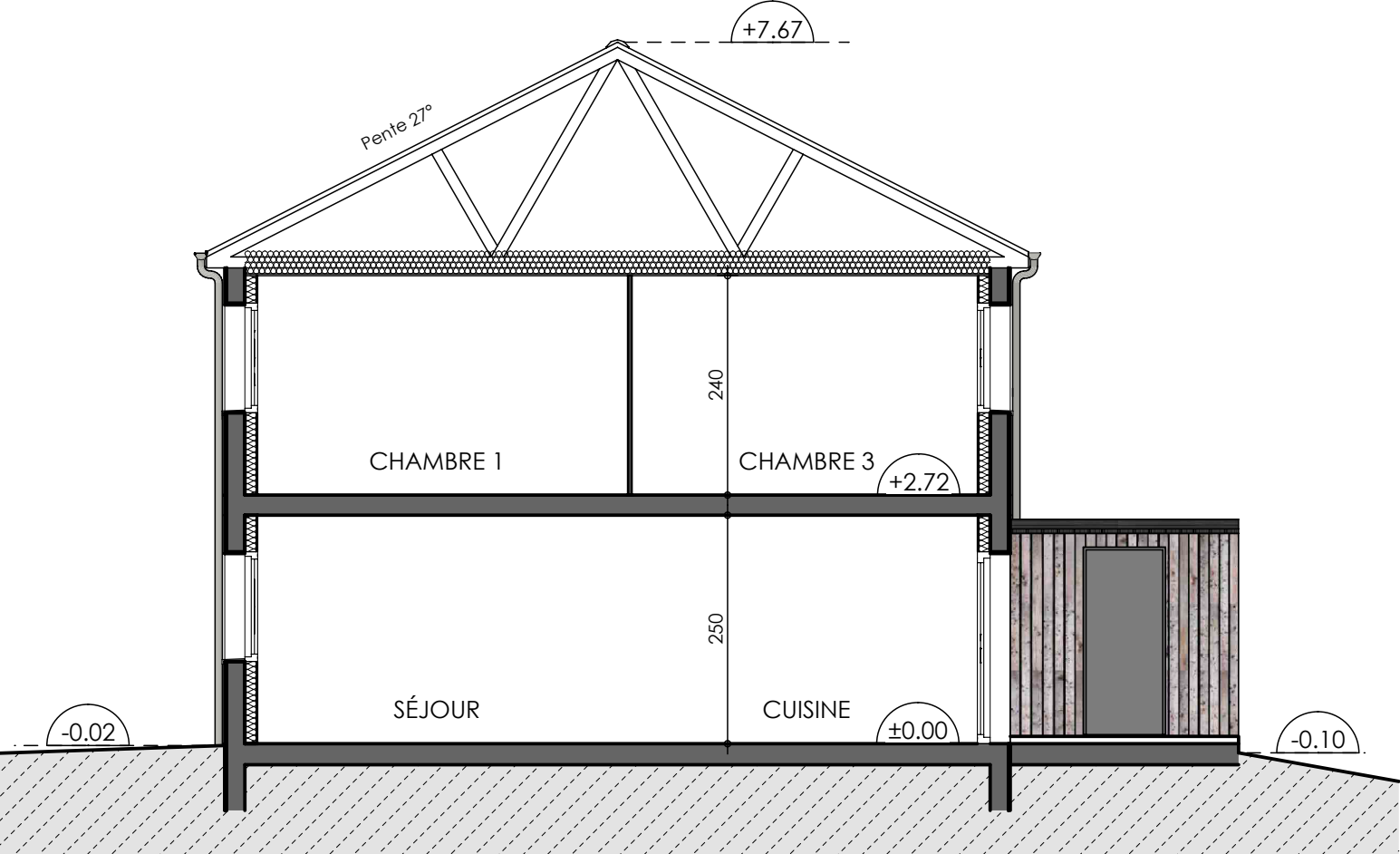
COUPE
